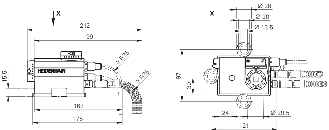
含固定夹、电缆和压缩空气管的视图
