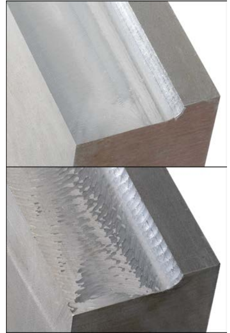
上图：用ACC功能铣削的零件 下图：未用ACC功能铣削的零件
