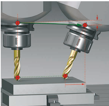
端面铣削
